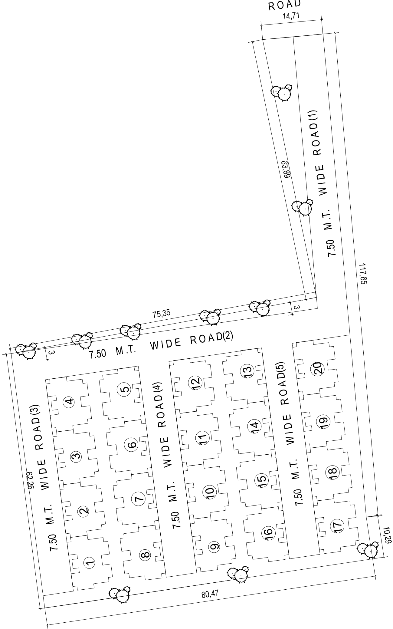
LAY-OUT OF AT T.P.NO-2,(UDHANA) F.P. NO.-95 PAIKI
